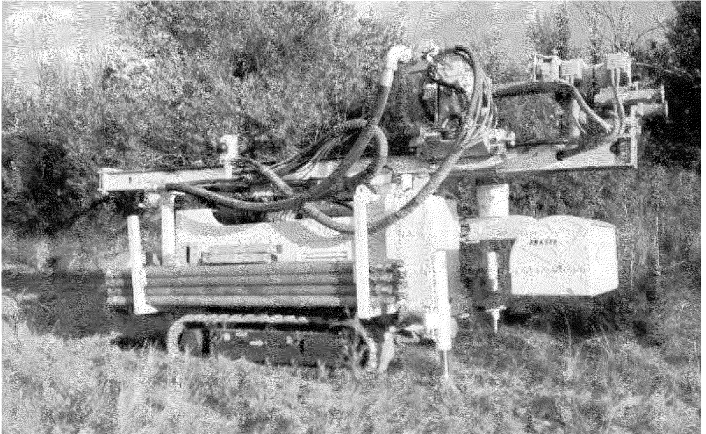
Un macchinario per la ricerca geotermica nel Volterrano (Foto di repertorio)
